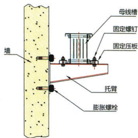
图2 水平墙装示意图
