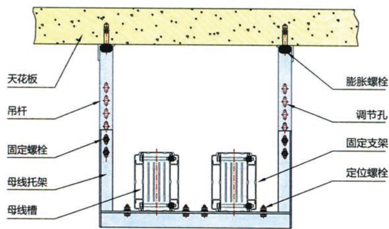
图1 双母线吊装示意图
