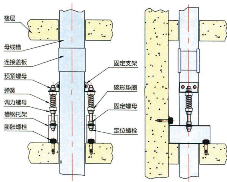
图3 垂直井道安装示意图
